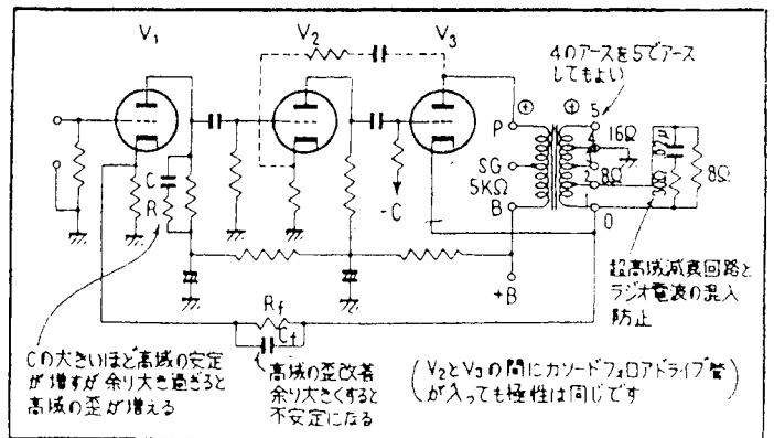
3段アンプのNFBとカソードNF
