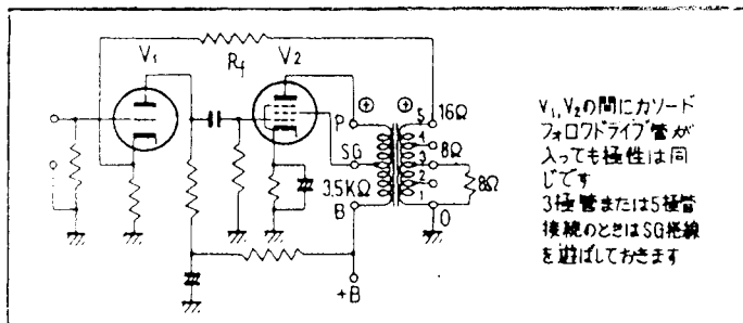
2段アンプのNFBとUL接続
