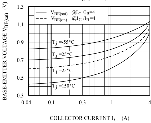
V_{BE(sat)} - I_C
