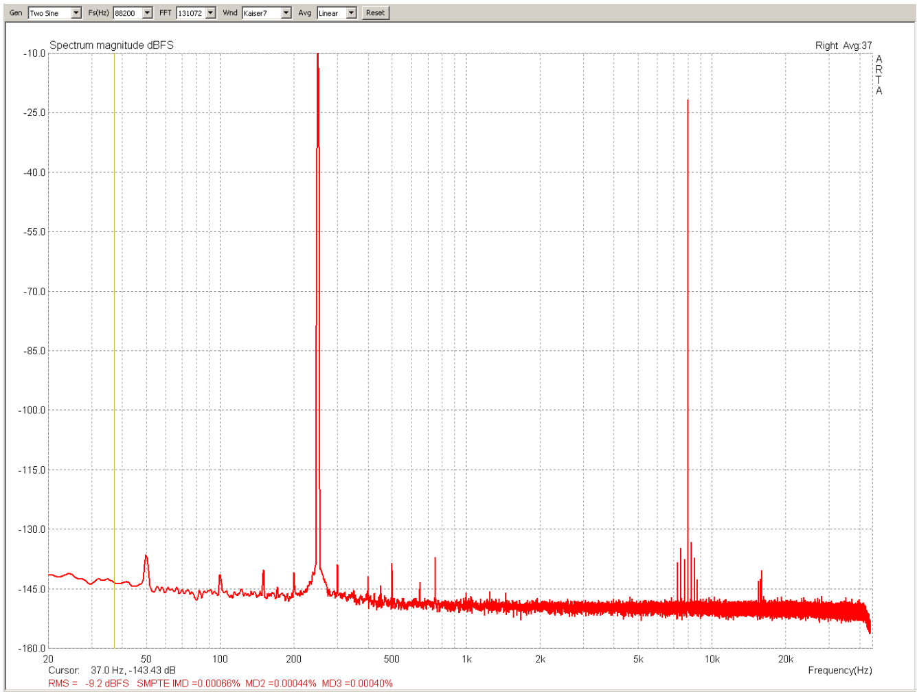
FE -V7 – 5W – SMPTE IMD
