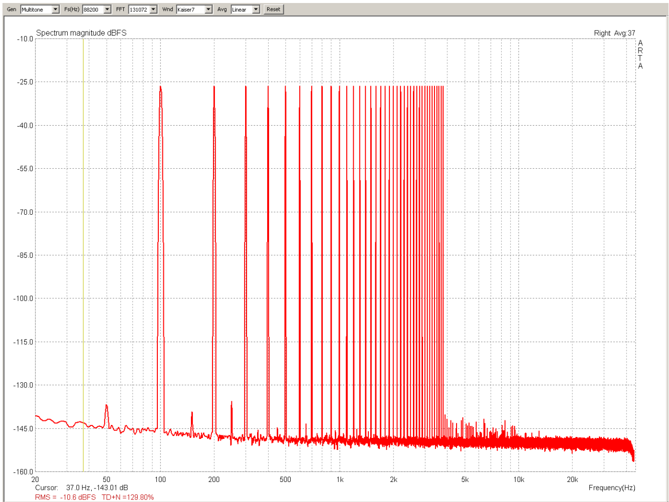
FE -V7 – 5W- ITU std. Multitone test
