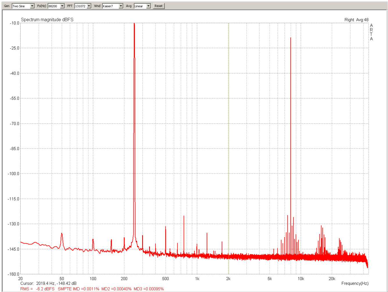
FE - V7 - 18W - SMPTE IMD
