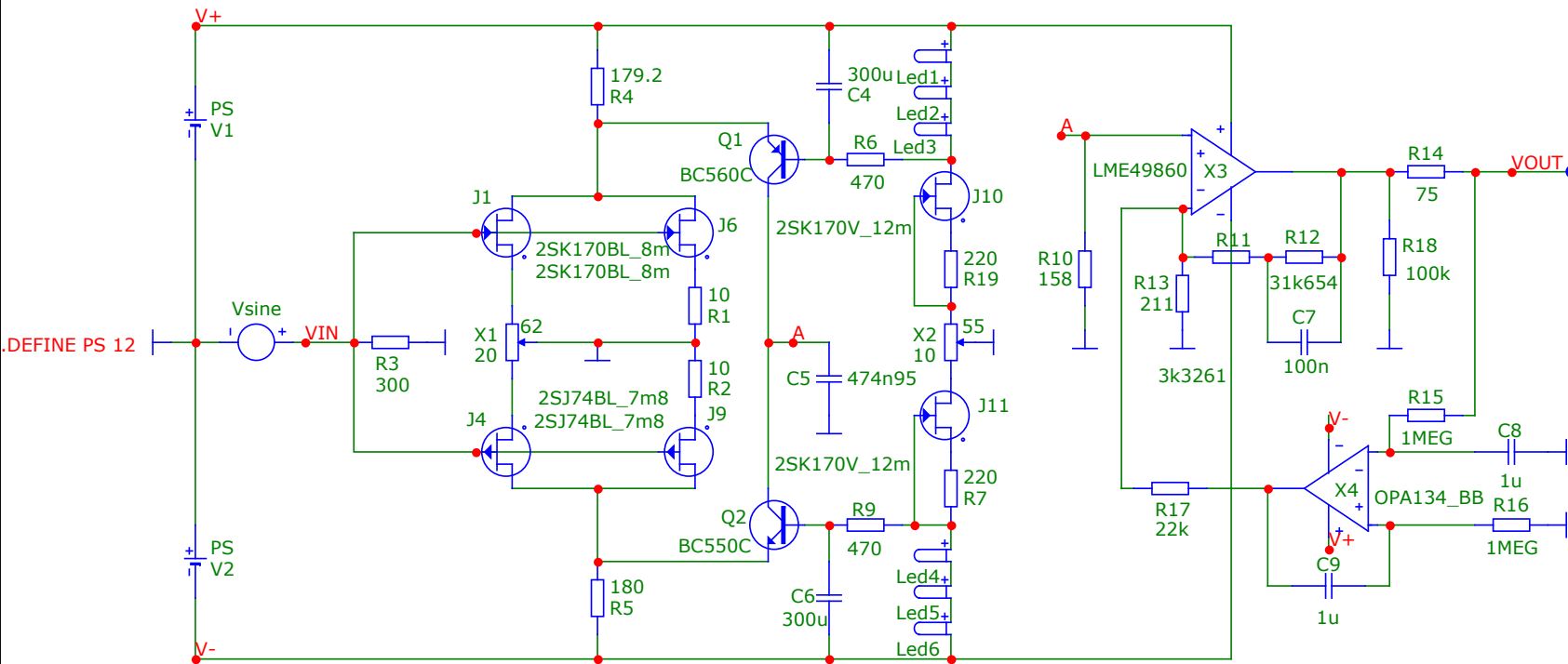
High Z MPP FET DC Offset Fine Adjust CPCitve RIAA REV B.cir
