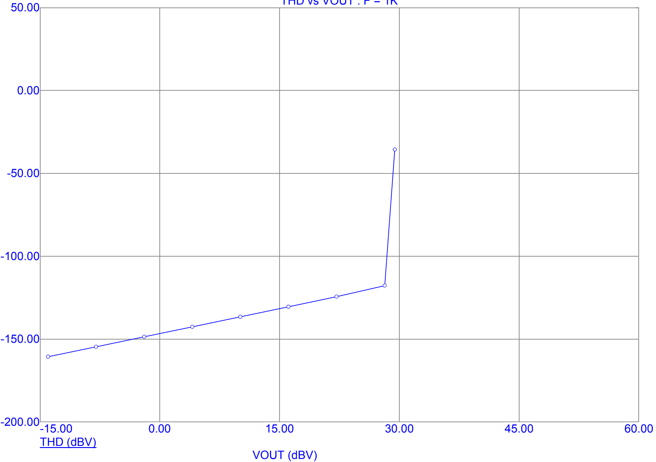
THD vs VOUT : F = 1K
