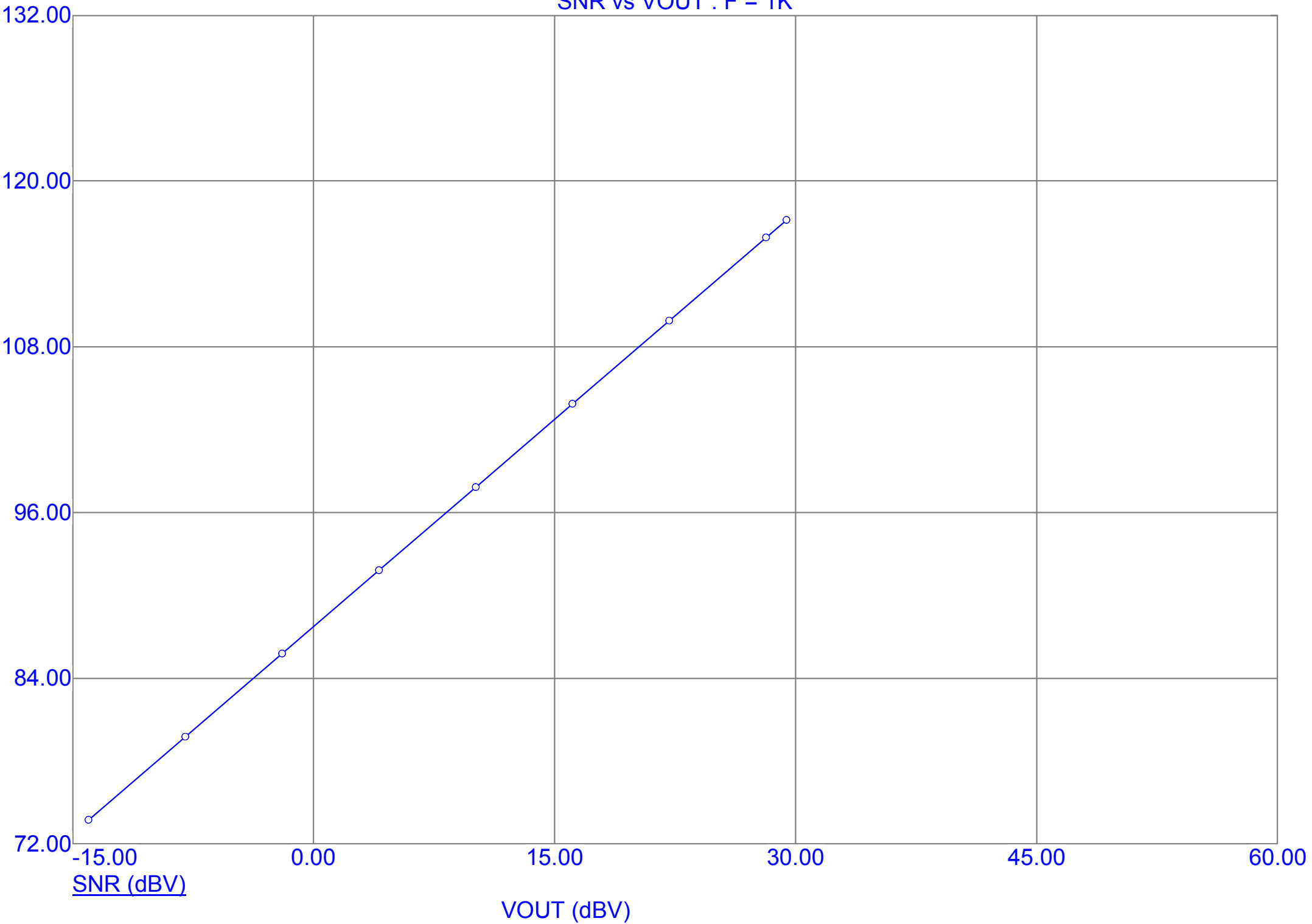
SNR vs VOUT : F = 1K
